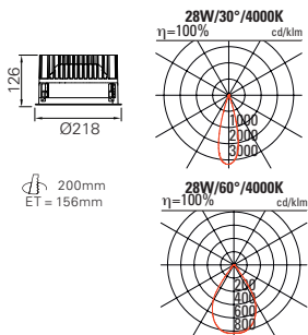
TAKEO T200 ohne Betriebsgerät (700mA)
